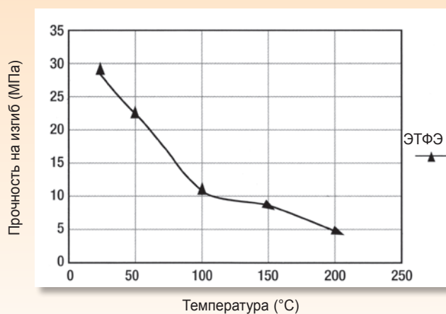
Влияние температуры на прочность на изгиб
