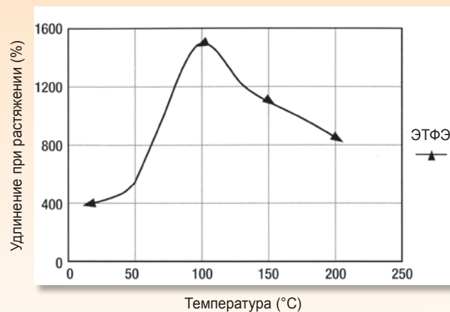
Влияние температуры на удлинение при растяжении
