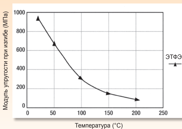
Влияние температуры на модуль упругости при изгибе
