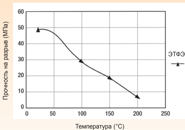
Влияние температуры на прочность на разрыв
